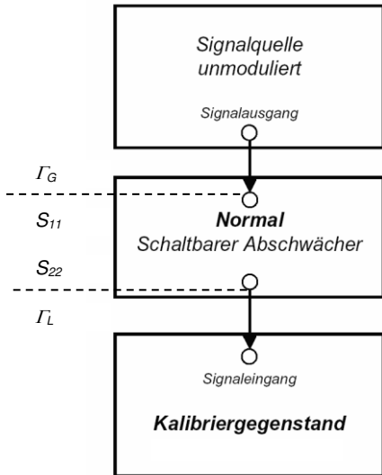
Bild XIII.5.6.1 Messaufbau Kalibrierung der Anzeigelinearität [7]
